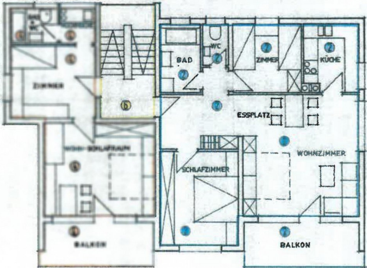
Grundriss
