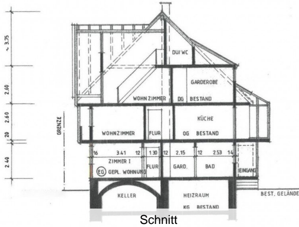
SCHNITT A-A
