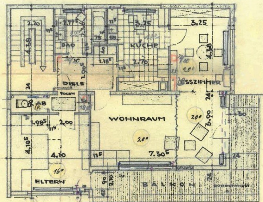
Grundriss Erdgeschoss
