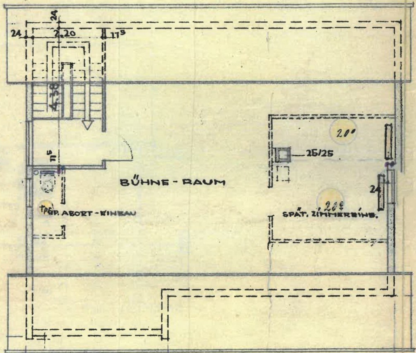
Grundriss Dachgeschoss
